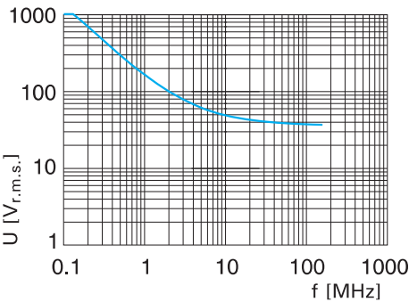
Spannung Schirm / Erde
