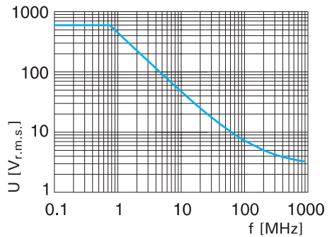
Spannung Innenleiter / Schirm
